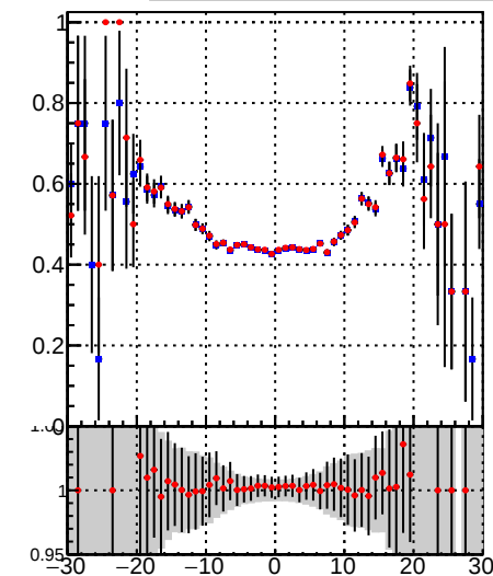
— Orig/DQM_orig_MS — pixelLessOrig/DQM_mod_MS
