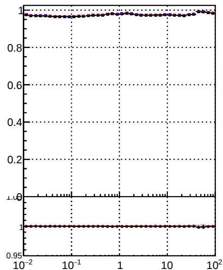
Fake rate vs v —•— Orig/DQM_orig_MS —•— pixelLessOrig/DQM_mod_MS —•— pixelLess/DQM_mod_MS
