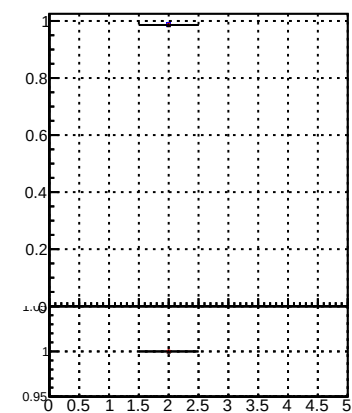
Orig/DQM_orig_MS pixelLessOrig/DQM_mod_MS pixelLess/DQM_mod_MS
