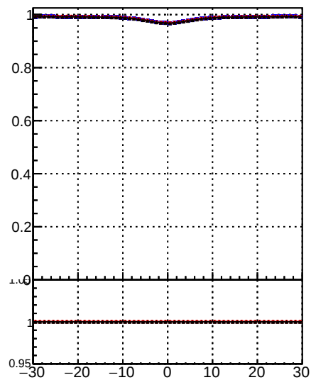
Fake rate vs d — Orig/DQM_orig_MS — pixelLessOrig/DQM_mod_MS — pixelLess/DQM_mod_MS
