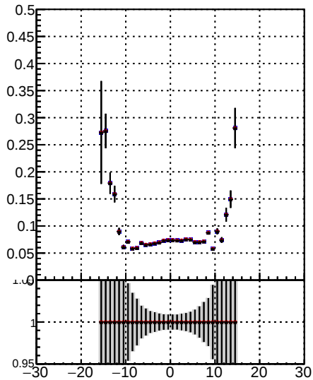
Fake rate vs d — Orig/DQM orig_MS — pixelLess/DQM orig_MS — pixelLess/DQM mod_MS
