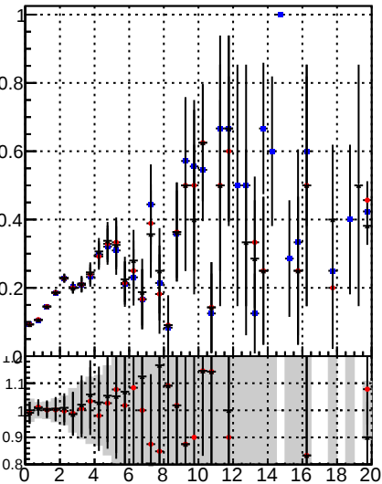
Fake rate vs. — Orig/DQM_orig_MS — Less/DQM_mod_MS — Pixel/DQM_mod_MS
