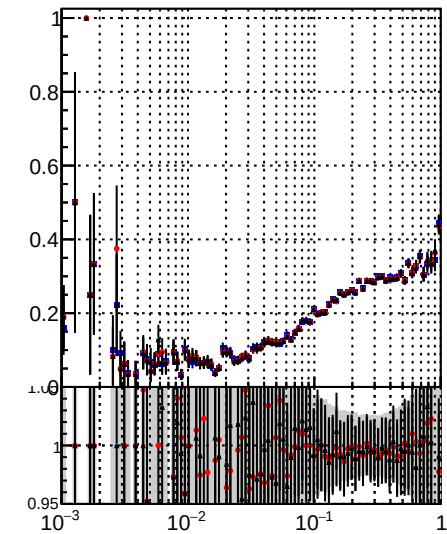
Fake rate vs dr —●— Orig/DQM orig_MS —●— pixelLessOrig/DQM_mod_MS —●— pixelLess/DQM_mod_MS
