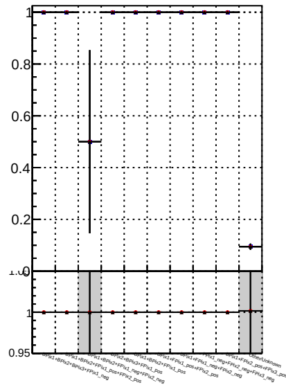
Fake rate vs. — Orig/DQM orig_MS — pixelLess/DQM orig_MS — pixelLess/DQM mod_MS
