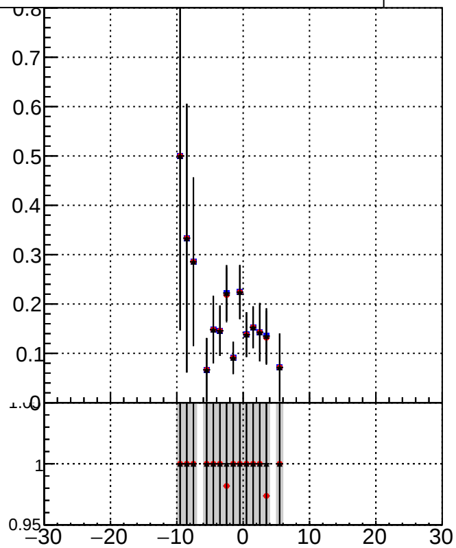
Orig/DQM_orig_MS pixelLessOrig/DQM_mod_MS pixelLess/DQM_mod_MS
