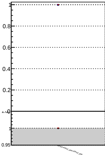
Fake rate vs. —•— Orig/DQM_orig_MS —•— pixelLessOrig/DQM_mod_MS —•— pixelLess/DQM_mod_MS
