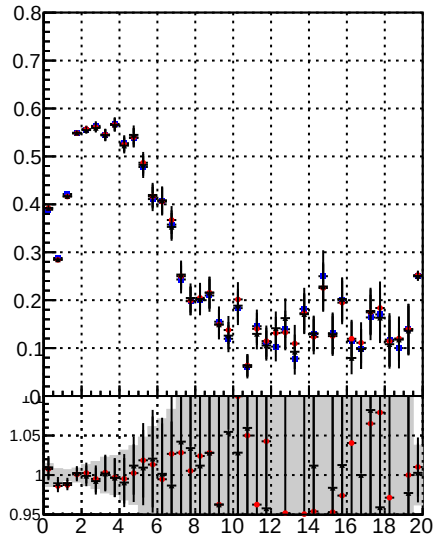
Fake rate vs. —●— Orig/DQM orig_MS —●— PixelLess/DQM mod_MS —●— Orig/DQM mod_MS
