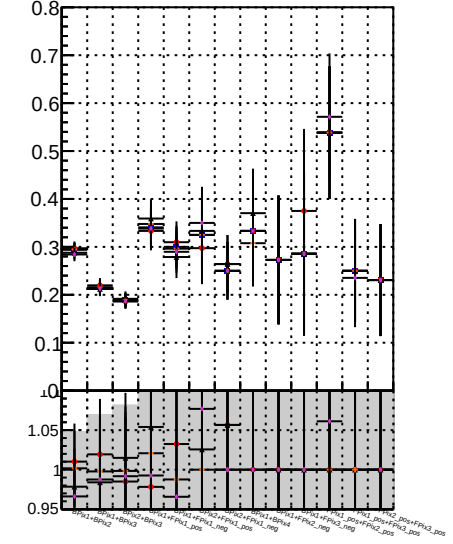
Fake rate vs. Orig/DQM orig MS Minus DQM orig MS Minus DQM orig MS Detached DQM orig MS
