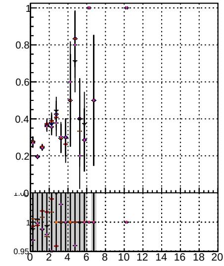
Fake rate vs. Orig/DQM orig MS Minus DQM orig MS Minus DQM orig MS Detached DQM orig MS
