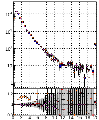
N of reco track vs. s Orig/DOM-orig-MS detached/DOM-orig-MS nbody/DOM-orig-MS nbody/DOM-orig-MS
