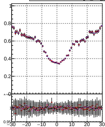
— Orig/DQM_orig_MS — DQM_orig_MS — DQM_orig_MS — detached/DQM_orig_MS
