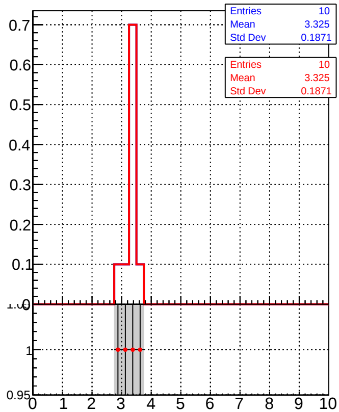
dE/dx estimator 1
