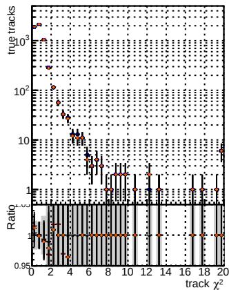
chi2 pdf
