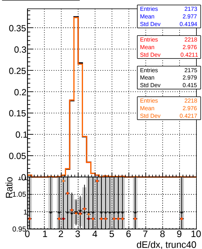
dE/dx estimator 2
