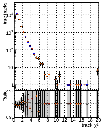
chi2 pdq
