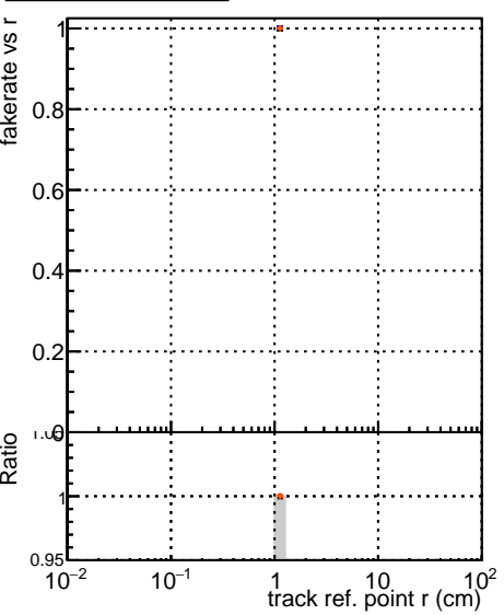
—•— DQM mkFit TToriginal —•— DQM mkFit TTNEW50_chi2 —•— DQM mkFit TTNEW50_apdq
