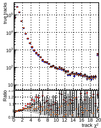
dpdq chi2
