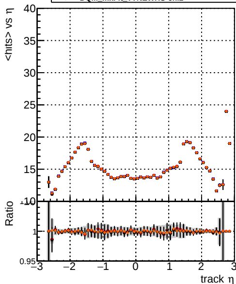
DQM_mkFit_TToriginal DQM_mkFit_TTNEUHS DQM_mkFit_TTNEUHS-dpdq DQM_mkFit_TTNEUHS-chi2 mean hits
