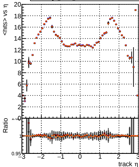
DQM_mkFit_TToriginal DQM_mkFit_TTNEUHS DQM_mkFit_TTNEUHS-dpdq DQM_mkFit_TTNEUHS-chi2 mean hit
