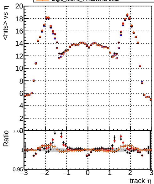
mean hit DQM_mkFit_TToriginal DQM_mkFit_TTNEUHS DQM_mkFit_TTNEUHS-dpdq DQM_mkFit_TTNEUHS-chi2
