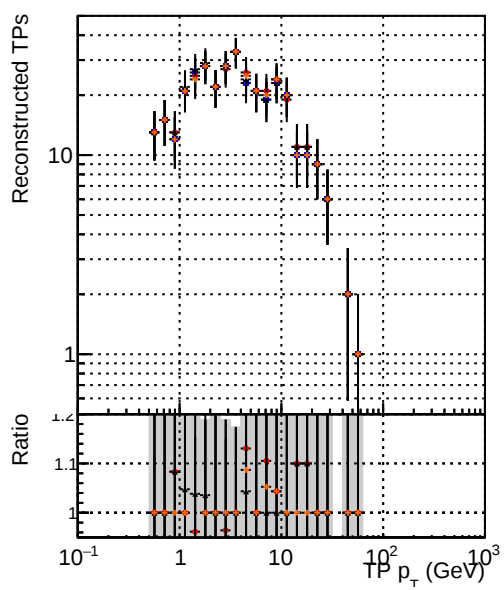
—•— DQM_mkFit_TToriginal —•— DQM_mkFit_TTNEUHS —•— DQM_mkFit_TTNEUHS-dpdq —•— DQM_mkFit_TTNEUHS-chi2
