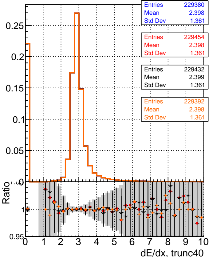
dE/dx estimator 2
