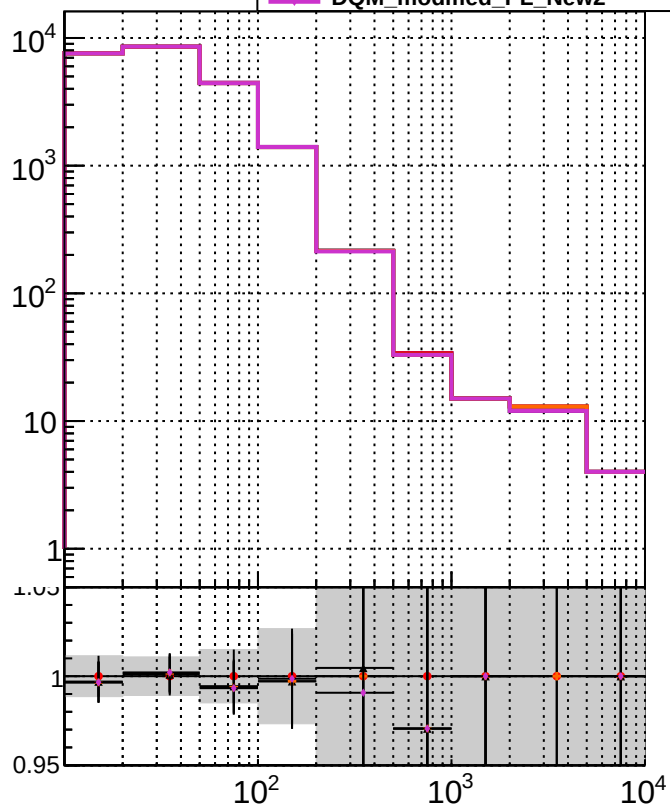
RecoAssoc2GenPVM
