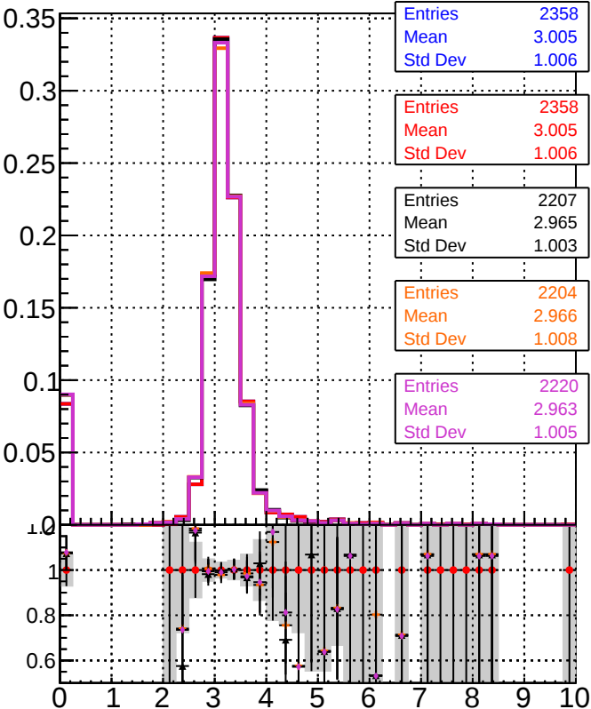
dE/dx estimator 1
