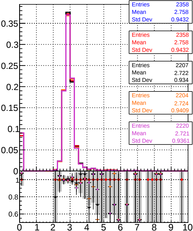
dE/dx estimator 2
