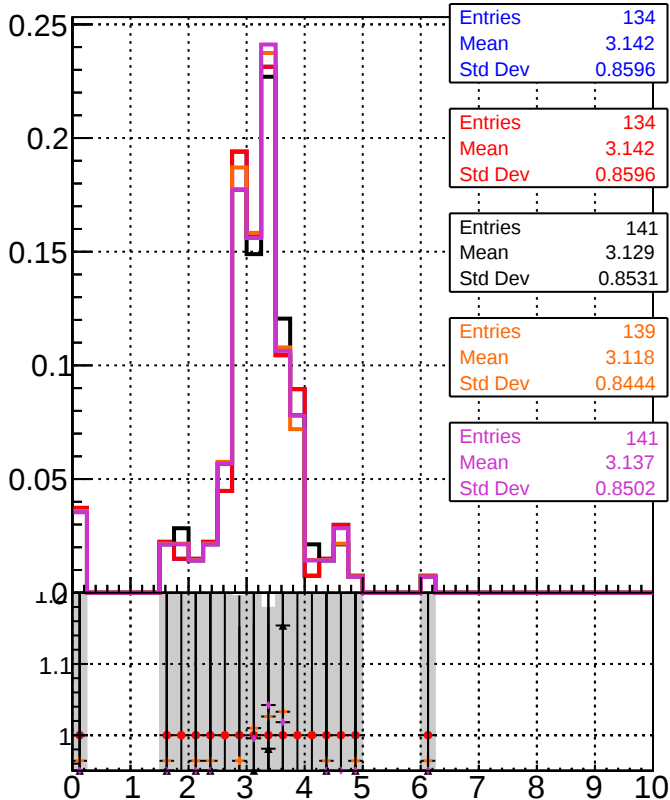
dE/dx estimator 1
