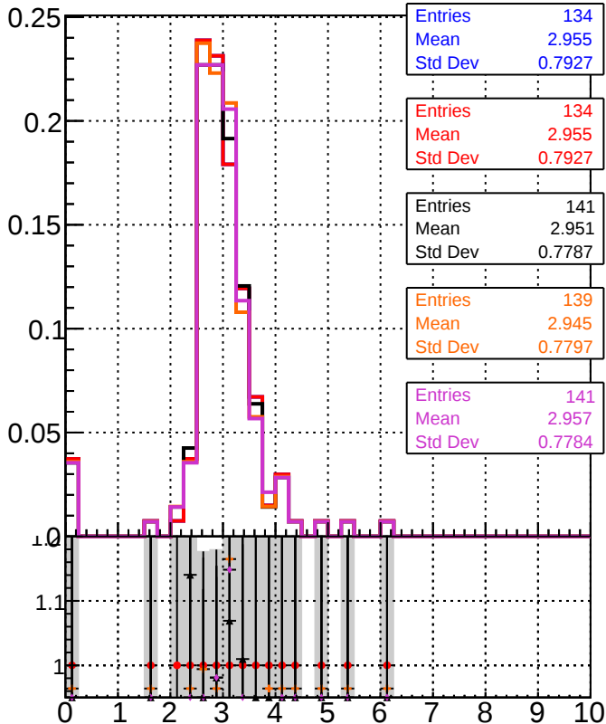
dE/dx estimator 2
