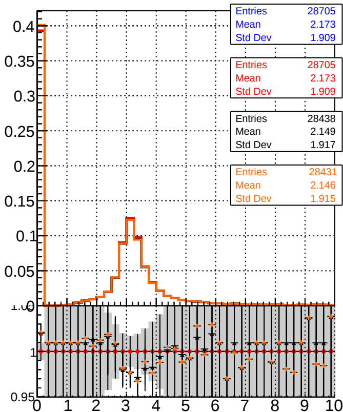
dE/dx estimator 1
