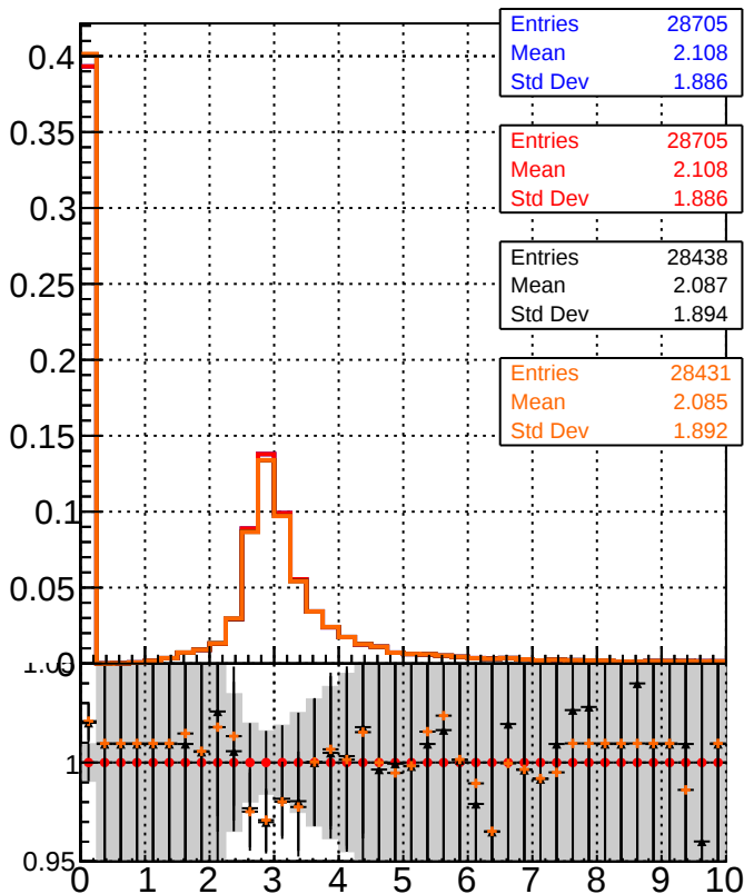
dE/dx estimator 2
