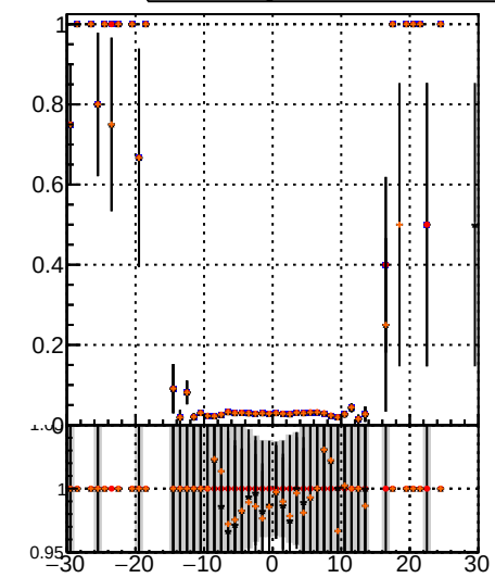
Fake rate vs vertpos DQM modified PL New1 DQM modified PL New1 DQM modified PL New1
