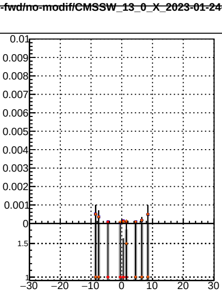
Fake rate vs vertpos DQM modified PL New1 DQM modified PL New1 DQM modified PL New1
