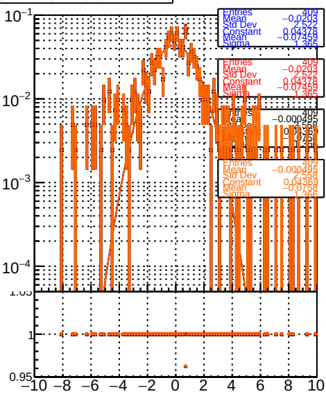
pull of q_{over} parameter
