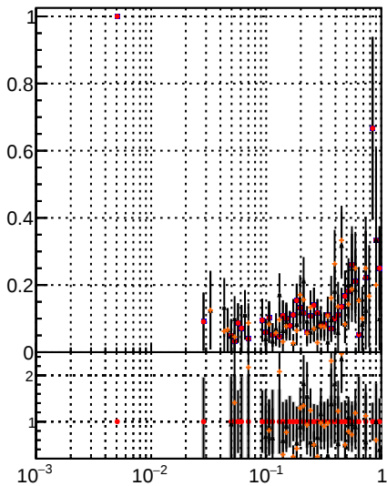
Fake rate vs dr DQM modified PL DQM modified PL New1 DQM modified PL New2 DQM modified PL New3
