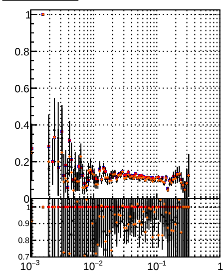
Fake rate vs dr DQM modified PL DQM modified PL New1
