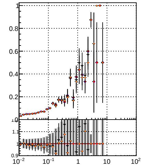
Fake rate vs \sqrt{s} DQM modified PL New1 DQM modified PL New1 DQM modified PL New1 DQM modified PL New1
