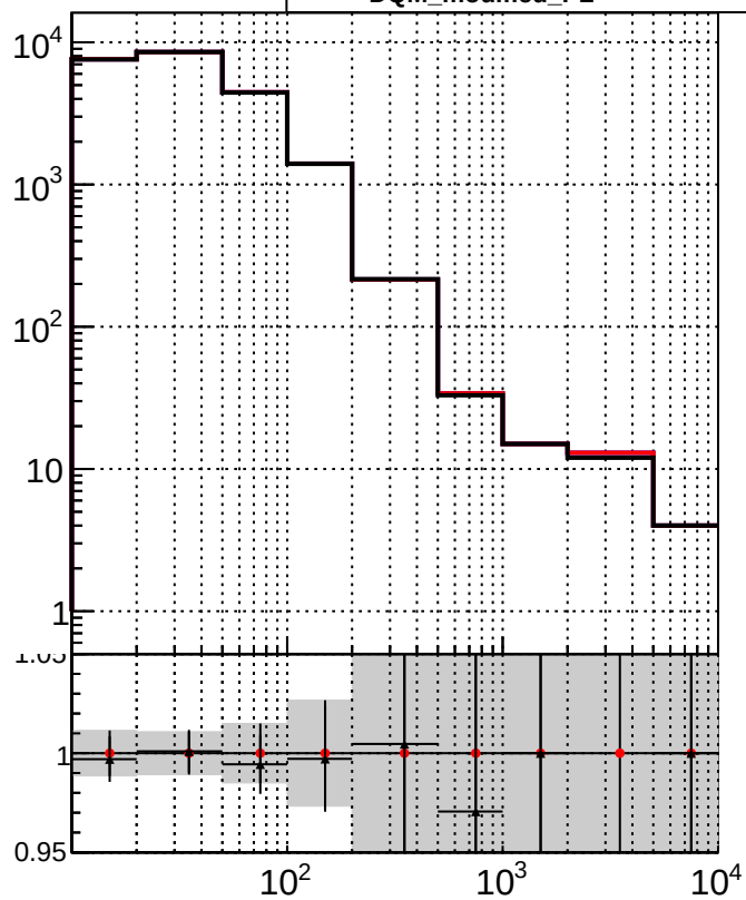
RecoAssoc2GenPV
