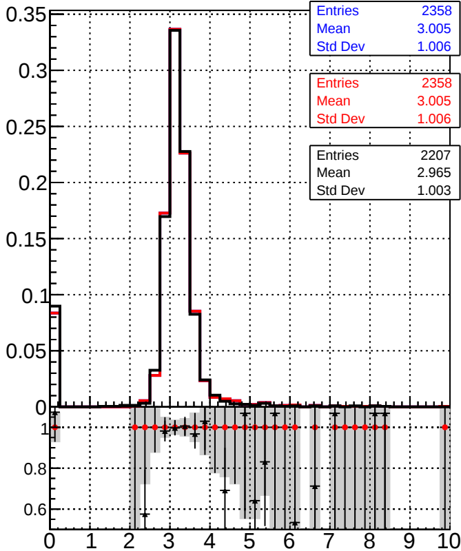
dE/dx estimator 1
