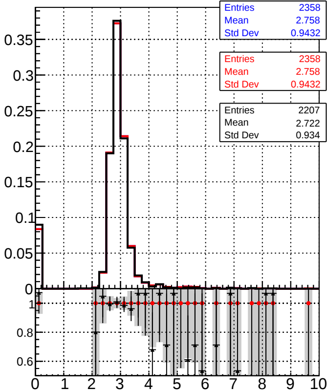
dE/dx estimator 2
