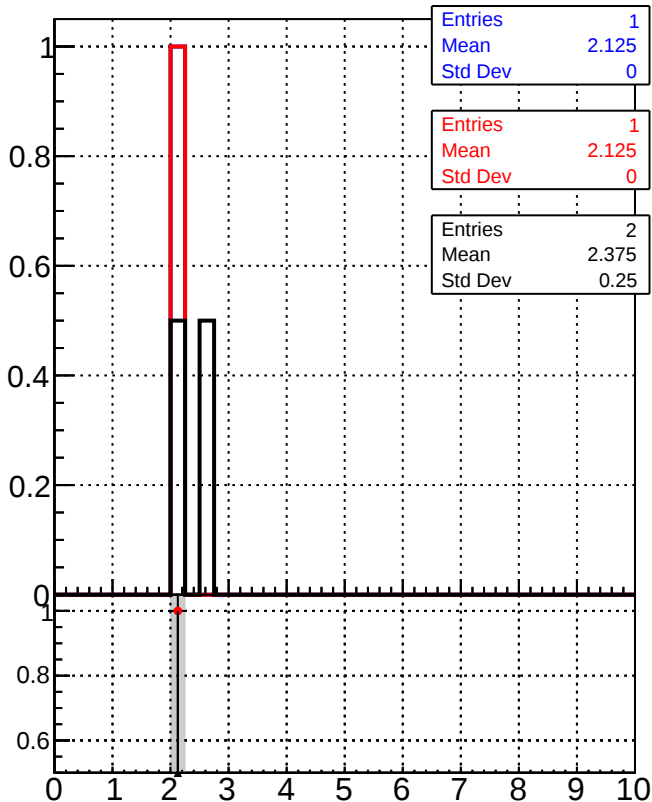
dE/dx estimator 1
