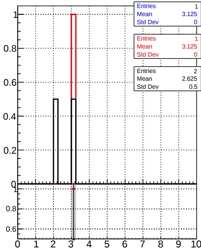
dE/dx estimator 2
