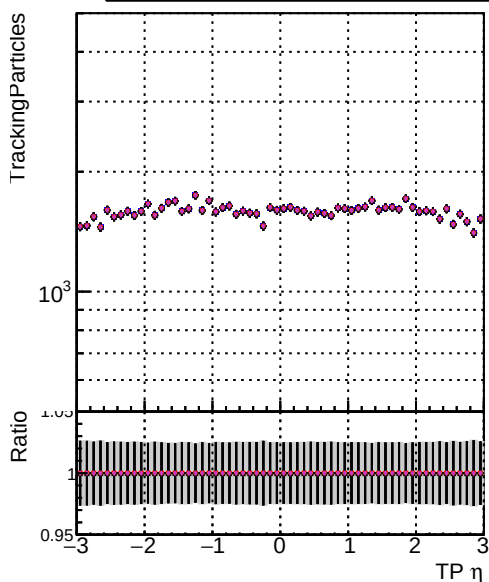
N of sin Legend DOM mkFit TT JanU Update-statErr ▲ DOM mkFit TT JanU Update-systErr + DOM mkFit TT JanU Update-bothErr + DOM mkFit TT JanU Update-systErr + DOM mkFit TT JanU Update-bothErr
