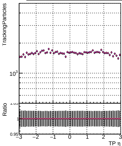
N of sin ▲ DOM mkFit TT JanU update-statErr + DOM mkFit TT JanU update-systErr + DOM mkFit TT JanU update-bothErr
