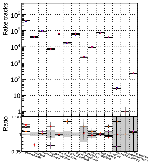
Number DOM mkFit TT JanUpdate-statErr DOM mkFit TT JanUpdate-statErr DOM mkFit TT JanUpdate-systErr DOM mkFit TT JanUpdate-bothErr
