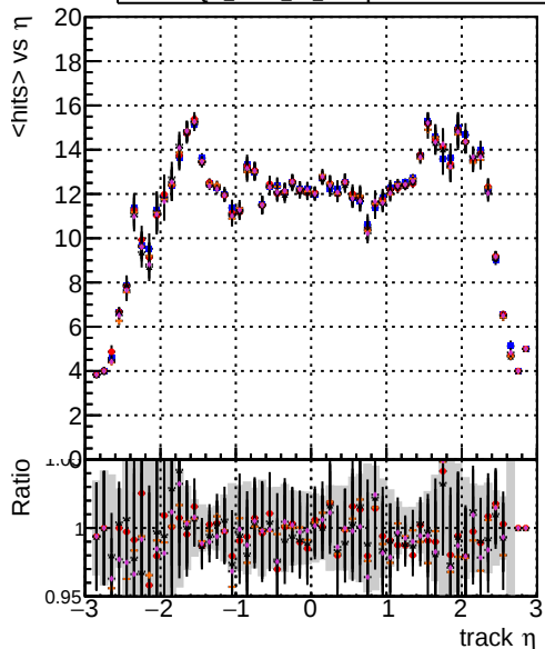
Legend: DQM mkFit TT original, DQM mkFit TT JanUpdate-noErr, DQM mkFit TT JanUpdate-statErr, DQM mkFit TT JanUpdate-systErr, DQM mkFit TT JanUpdate-bothErr mean hit
