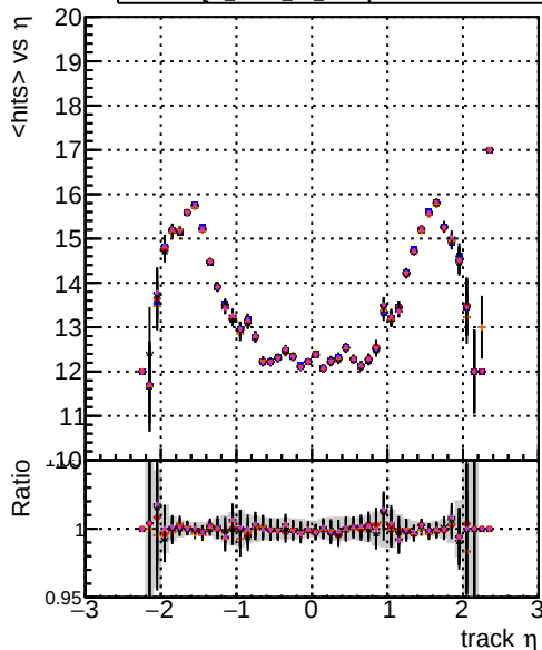
mean hit DQM mkFit 11 original DQM mkFit 11 JanUpdate-noErr DQM mkFit 11 JanUpdate-statErr DQM mkFit 11 JanUpdate-systErr DQM mkFit 11 JanUpdate-bothErr
