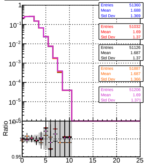
mean hit DQM mkFit 11 original DQM mkFit 11 JanUpdate-noErr DQM mkFit 11 JanUpdate-statErr DQM mkFit 11 JanUpdate-systErr DQM mkFit 11 JanUpdate-bothErr
