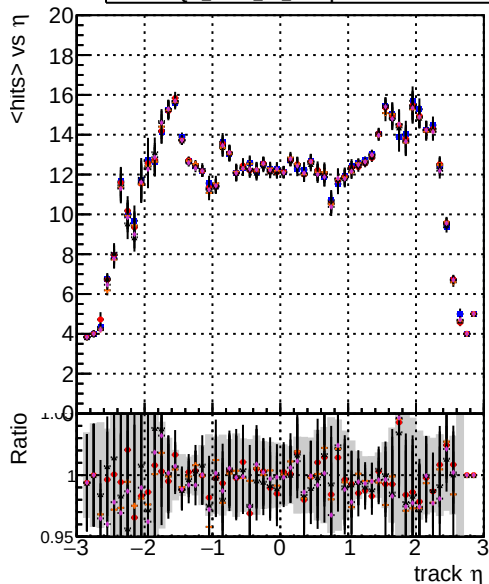
Legend for mean hits vs \eta : DOM mkFit TT original DOM mkFit TT JanUpdate-noErr DOM mkFit TT JanUpdate-statErr DOM mkFit TT JanUpdate-systErr DOM mkFit TT JanUpdate-bothErr
