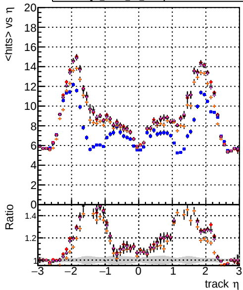
mean hit DQM mkFit TT original DQM mkFit TT JanUpdate-noErr DQM mkFit TT JanUpdate-statErr DQM mkFit TT JanUpdate-systErr DQM mkFit TT JanUpdate-bothErr
