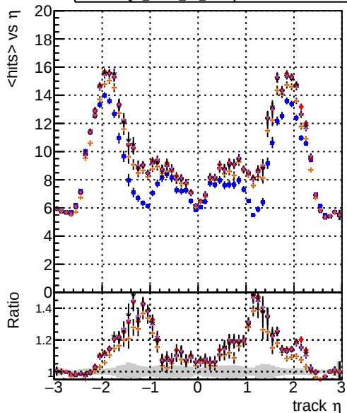
Legend: DQM mkFit TT original, DQM mkFit TT JanUpdate-noErr, DQM mkFit TT JanUpdate-statErr, DQM mkFit TT JanUpdate-systErr, DQM mkFit TT JanUpdate-bothErr mean hits
