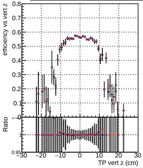
Efficiency vs. TP vert z (cm) DOM mkFit TT original DOM mkFit TT JanUpdate-noErr DOM mkFit TT JanUpdate-statErr DOM mkFit TT JanUpdate-systErr DOM mkFit TT JanUpdate-bothErr
