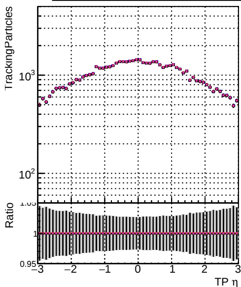
N of sin Model Fit TT JanU Update-statErr 1 DOM mkFit TT JanU Update-statErr 2 DOM mkFit TT JanU Update-systErr 3 DOM mkFit TT JanU Update-bothErr
