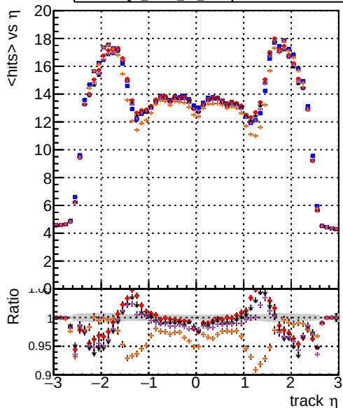
mean hit DOM mkFit TT JanUpdate-noErr DOM mkFit TT JanUpdate-statErr DOM mkFit TT JanUpdate-systErr DOM mkFit TT JanUpdate-bothErr
