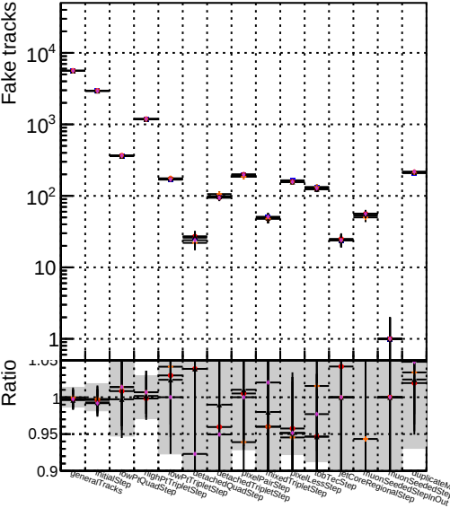
Number Symbol Label ▲ DQM_mkfFit_TT_JanUpdate-statErr ● DQM_mkfFit_TT_JanUpdate-systErr ▼ DQM_mkfFit_TT_JanUpdate-bothErr
