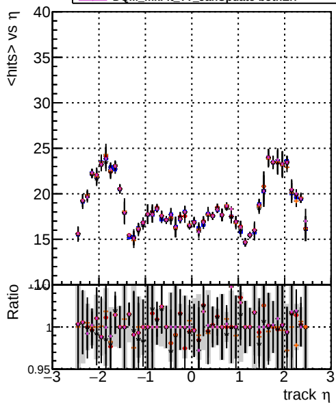
mean hits DOM mkFit TT JanUpdate-noErr DOM mkFit TT JanUpdate-statErr DOM mkFit TT JanUpdate-systErr DOM mkFit TT JanUpdate-bothErr
